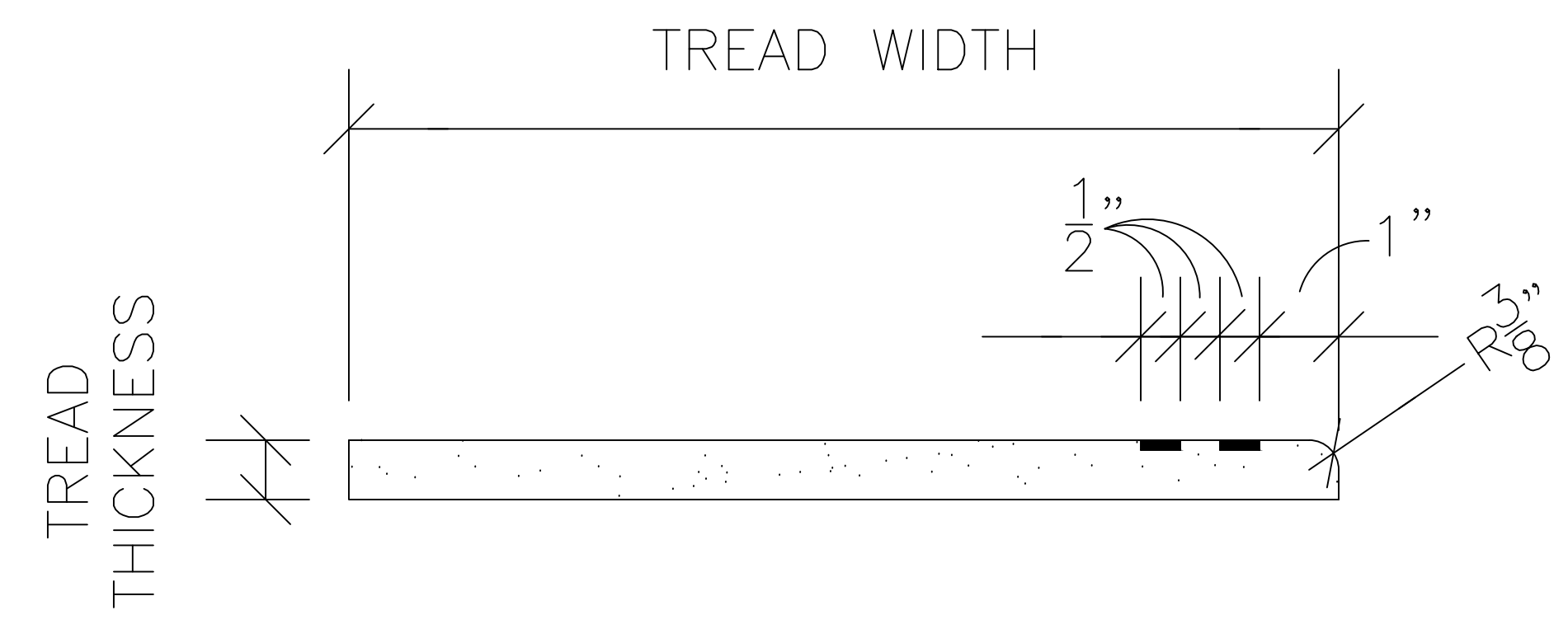
TREAD SECTION Scale: 6" = 1'-0"
