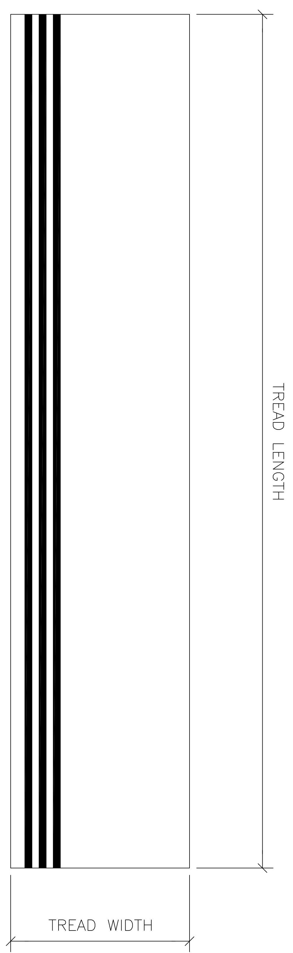
TERRAZZO TREAD PLAN VIEW SCALE: 3" = 1'-0"
